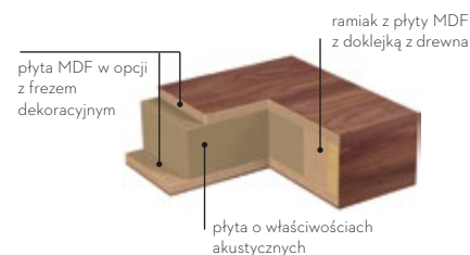
PRZEKRÓJ SKRZYDŁA ANDORA, BOLZANO
